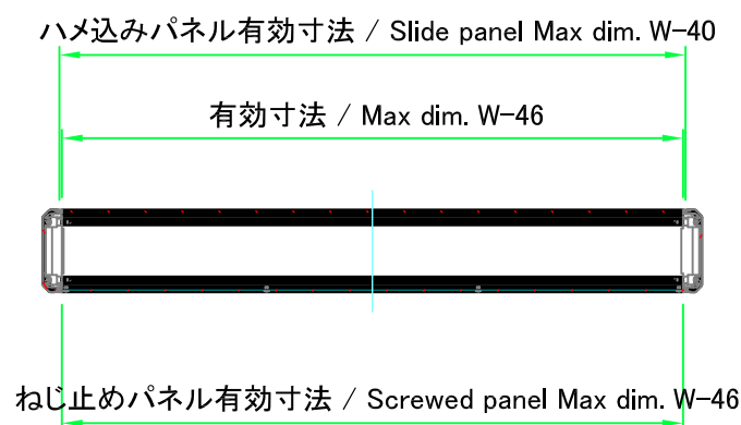
A-A ( 1 : 10 )
